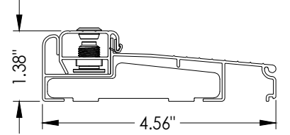
15 INSWING ADJUSTABLE THRESHOLD ZAILAA4565
